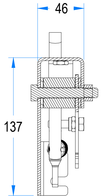
A-A Section
