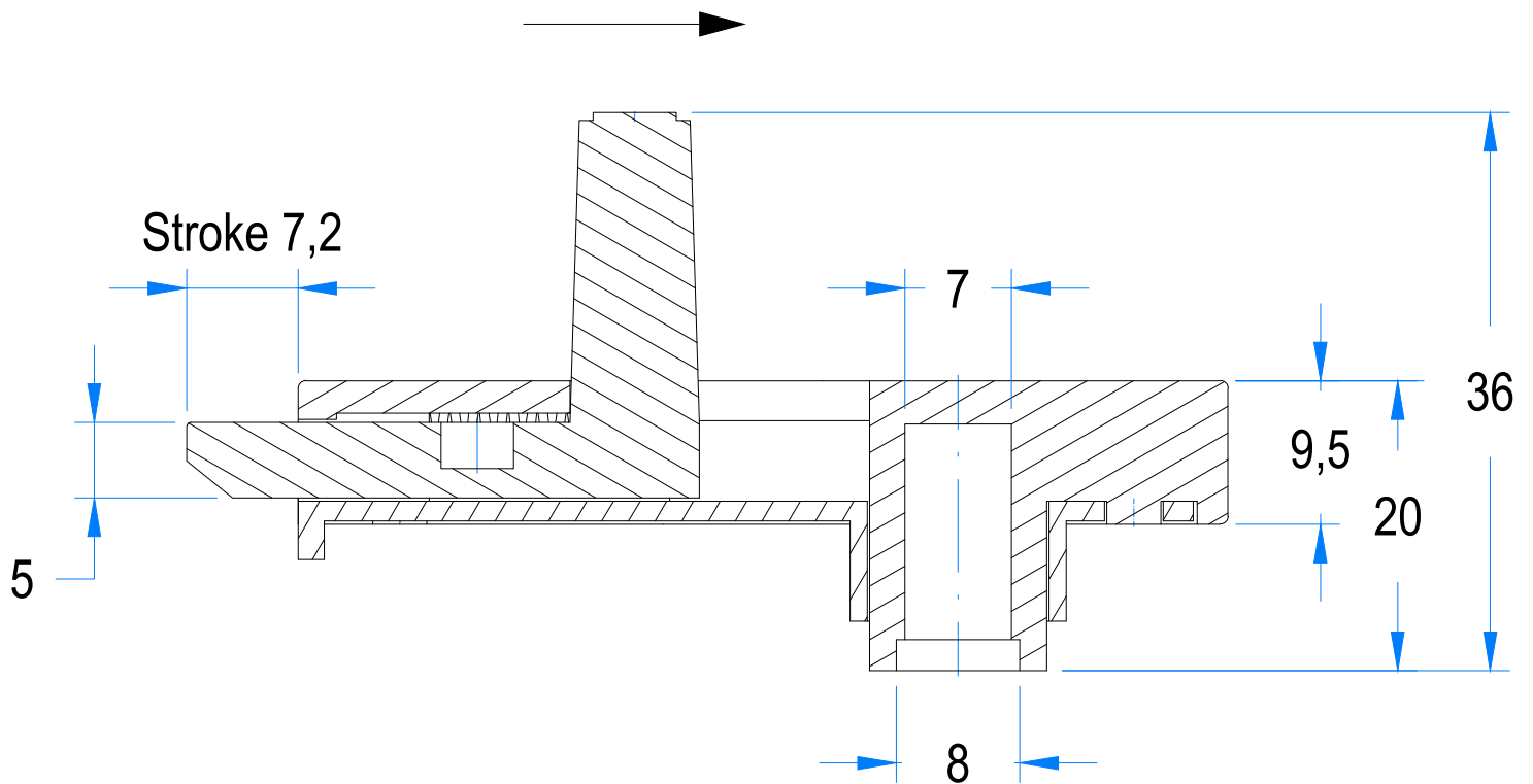
A-A Section
